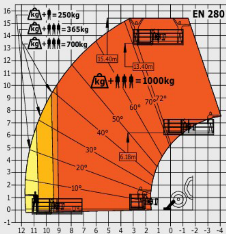
Maschine auf Stützen mit Arbeitsbühne (Versionen MT 1440 A und MT 1440 HA)
